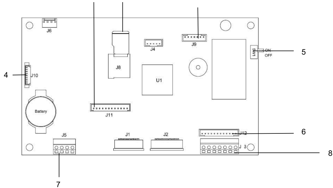
Abbildung 1-3 Hauptplatine
