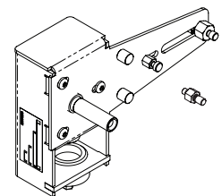
AV-611 SmartX Actuator Globe Linkage
